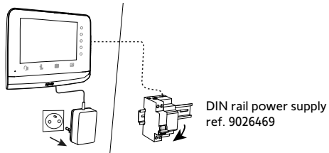
V@500
