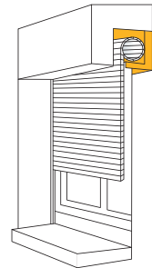
Coffre traditionnel
